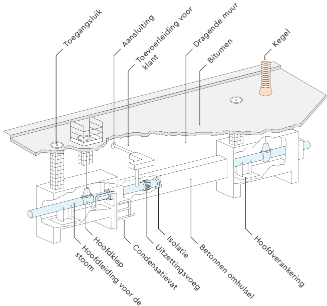
1/ NETWERK VAN PIJPLEIDINGEN
