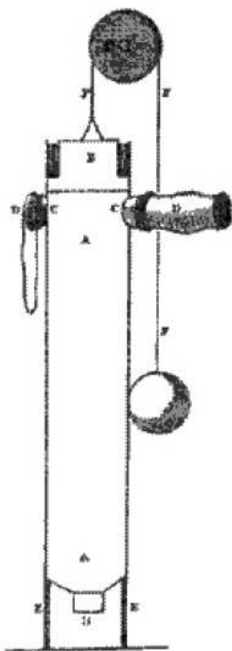
Buskruitmotor Christiaan Huygens
