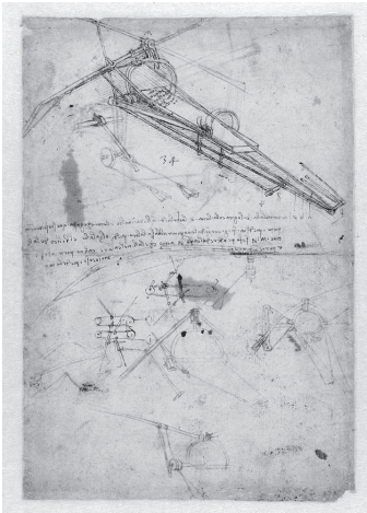
Da Vinci's schets van een 'vliegmachine' uit de Codex Atlanticus (1478-1519).
