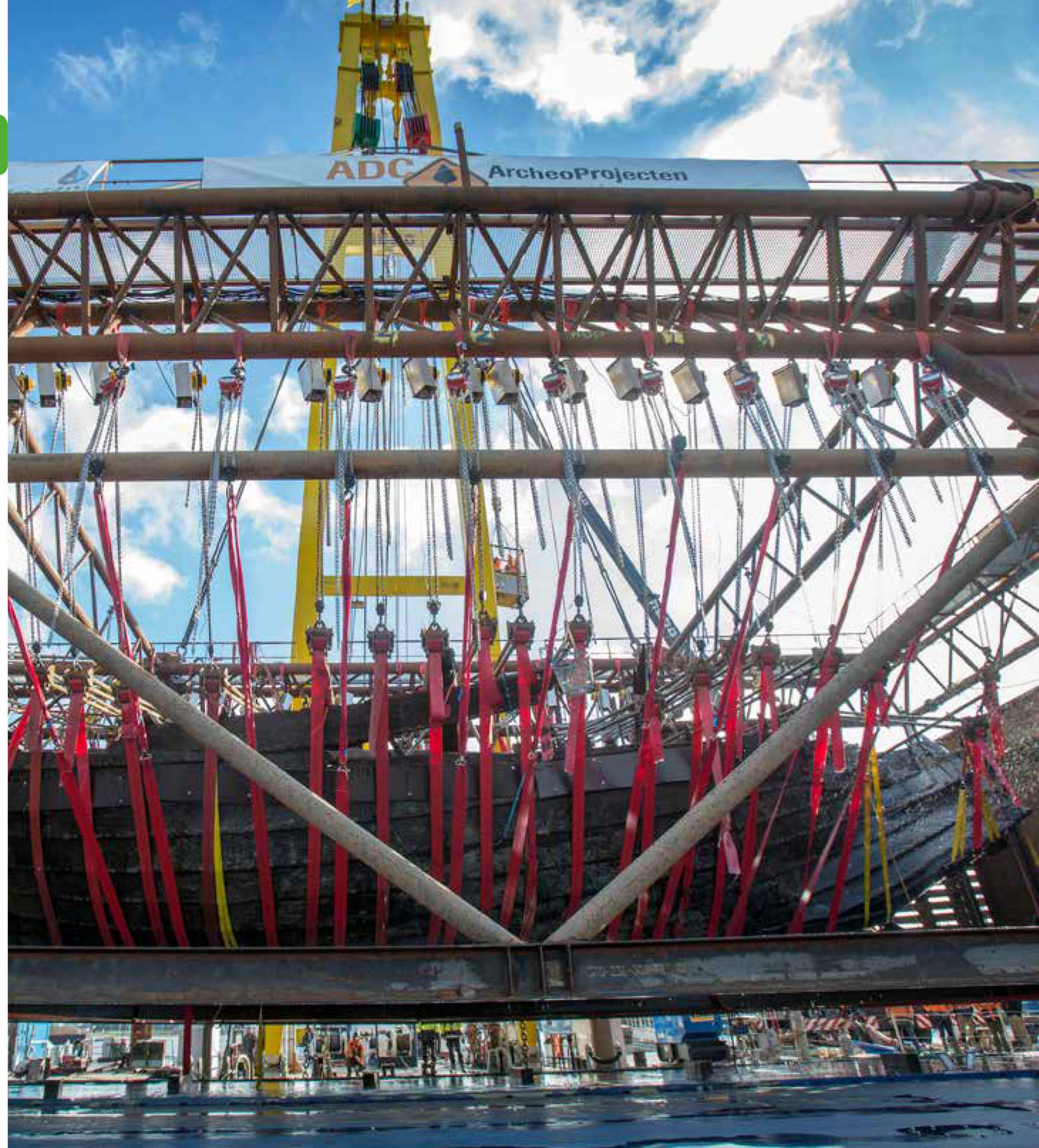
De kogge werd met schroeven en planken stevig gemaakt. Daarna werd er onder water een stalen kooi om het schip gebouwd. Met meer dan 100 sterke banden werd de kogge uit de IJssel getakeld.
